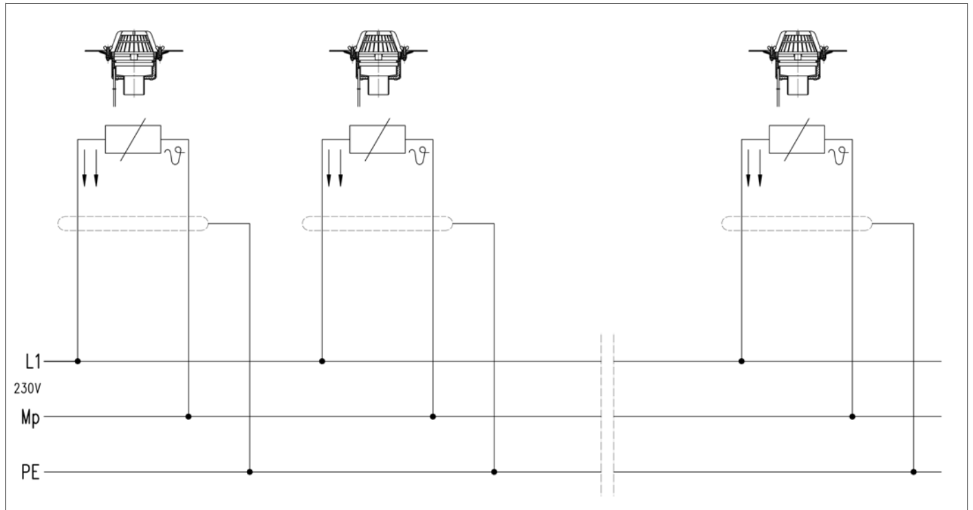
Figuur 10.61 Aansluitschema verwarming
